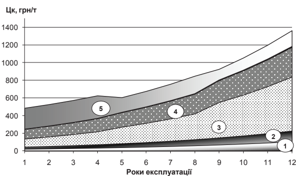
Рис. 2. Динаміка складових ціни концентрату за 1-м варіантом: 1 – витрати на видобуток руди, грн./т; 2 – витрати на дроблення руди, грн./т; 3 – витрати на розроблення 1мі породи розкриття, грн./мі; 4 – витрати на збагачення руди, грн./т; 5 – прибуток від реалізації концентрату, грн./т
