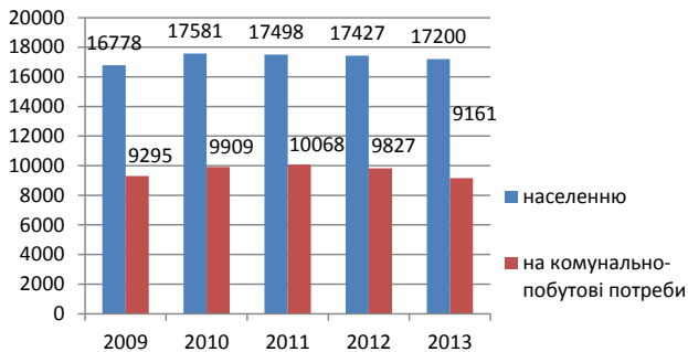
Рис. 5. Динаміка відпуску природного газу населенню та на комунально-побутові потреби за 2009–2013 рр., млн м 3 [4]
